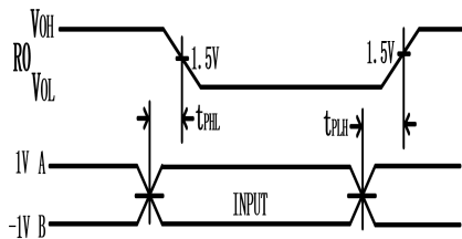
图 7 接收器传输延时
