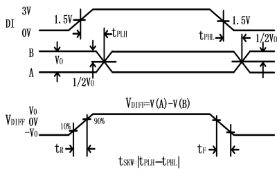
图 5 驱动器传输延时
