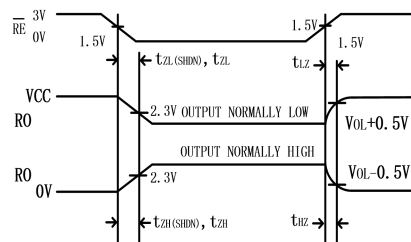
图 8 接收器使能/关断时序
