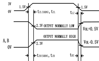
图 6 驱动器使能/关断时序
