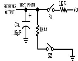
图 2 接收器使能/关断 开关特性测试负载
