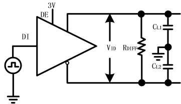
图 3 驱动器开关特性测试电路
