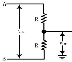
图 1 驱动器直流特性测试负载
