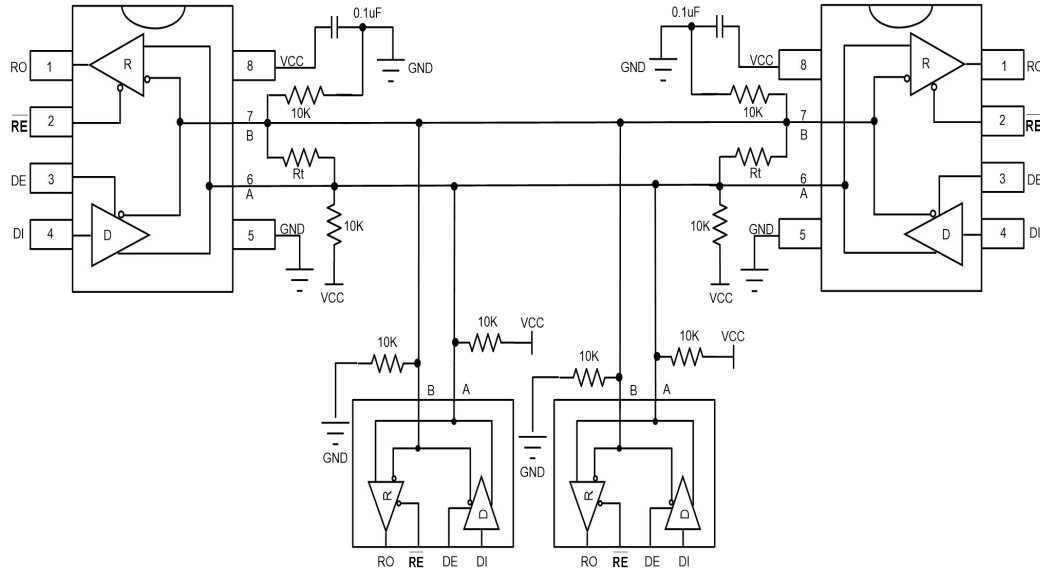
CN3485W 外围参考电路:
