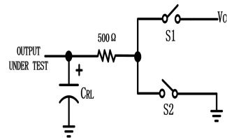
图 4 驱动器使能/关断 开关特性测试负载
