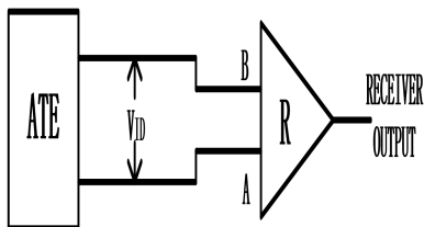
图 9 接收器传输延时测试电路
